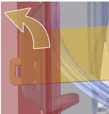
Abbildung 6: Hilfsrahmen-Klickmechanismus
