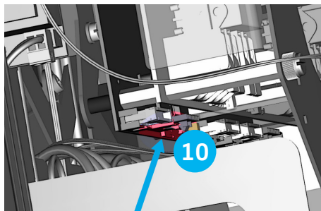
Abbildung 7: Position des SIM-Kartenhalters
