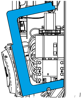
Abbildung 5: Abnehmbarer Hilfsrahmen
